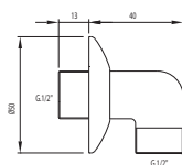
Codo toma pared para flexo Toma agua 1/2"
