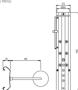
Columna de ducha termostática AVAN-TRES Ducha fija anticalcárea Ø 250 mm. Ducha móvil masaje. Pared o rincón. Fácil acceso a los filtros.
