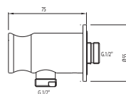
Soporte redondo para ducha LOFT con toma pared
