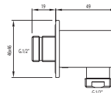
Codo toma pared para flexo Toma agua 1/2"
